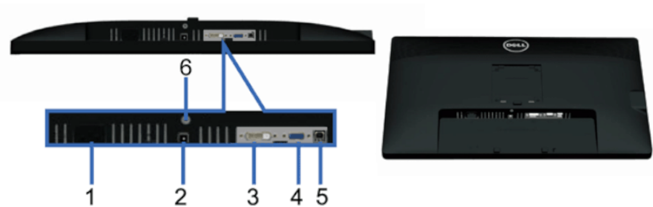
底视图
